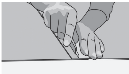
Рис. 38. Положить полотнища внахлест (3-5 см) и разрезать одновременно два полотнища по металлической планке.
