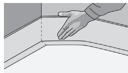
Рис. 47. Сделайте паз глубиной 2/3 от толщины плинтуса с обратной стороны, согните и поместите в угол. Затем прикатайте к стене с помощью специального ролика.
