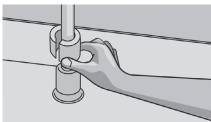
Рис. 71. 1. Прикрепите обшивку клеем рядом с трубой, сварите швы специальным феном. 2. Заранее подготовленная крышка приспособляется согласно инструкциям производителя. Можно использовать герметизирующий состав, подходящий для этих целей (силикон, Aquotat или подобный), чтобы лучше закрепить покрытие вокруг трубы. Используйте его между основанием и виниловым покрытием.
