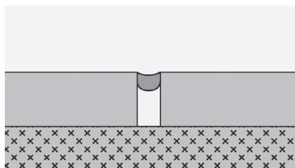
Рис. 33. Площадь контакта сварочного шнура и покрытия слишком маленькая: примерно 10-15 N/см.
