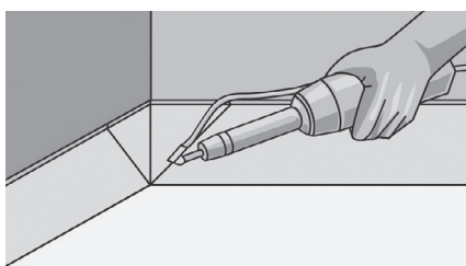
Рис. 69. Для соединения стыков используйте метод горячей сварки и необходимое оборудование.
