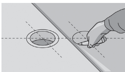
Рис. 72. Рядом с водосточной трубой, отогните покрытие от трубы. Сделайте пометку на покрытии, где находится середина трубы. Вырежьте на отогнутом покрытии отверстие. Нагрейте виниловое покрытие и прижмите его к трубе. Обрежьте излишки крючковым ножом так, чтобы стенки трубы были закрыты.
