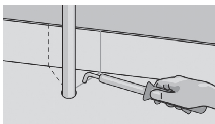
Рис. 70. При укладке напольного покрытия вокруг труб рядом со стенами, надрежьте покрытие и прижмите его к трубе, чтобы сформировать «воротник». Если расстояние между трубой и стеной маленькое, сделайте надрез так, чтобы потом осталась возможность его беспрепятственно сварить. Т.е. качество сварки и последующая функциональность имеют приоритет над эстетическим внешним видом.
