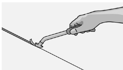
Рис. 27. Сделайте канавку резак.
