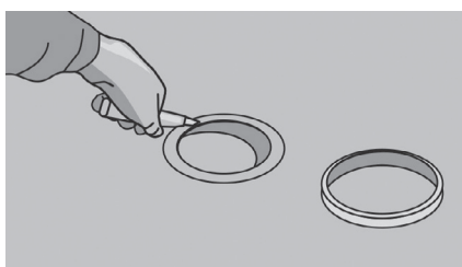
Рис. 73. Нагрейте покрытие рядом с открытым водостоком и отметьте расположение водостока с помощью зажимного кольца. Сделайте неболь-
