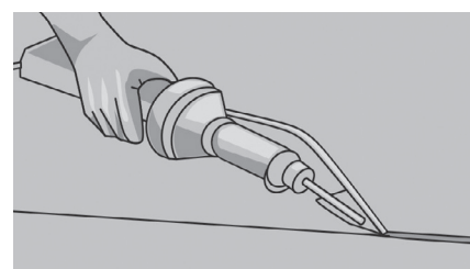
Рис. 75. Соедините шов методом горячей сварки с использованием скоростной насадки. Сварку можно производить через 24 часа после приклеивания.
