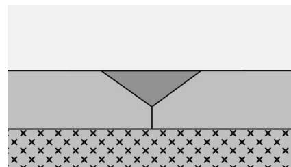
Рис. 31. Большая площадь контакта сварочного шнура и покрытия. При этом прочность сваренного шнура примерно 140 N/см.
