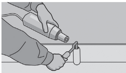
Рис. 92. Если настенное покрытие укладывается во влажной комнате, рекомендуем использовать фен, когда прижимаете покрытие к стене рядом с полом.
